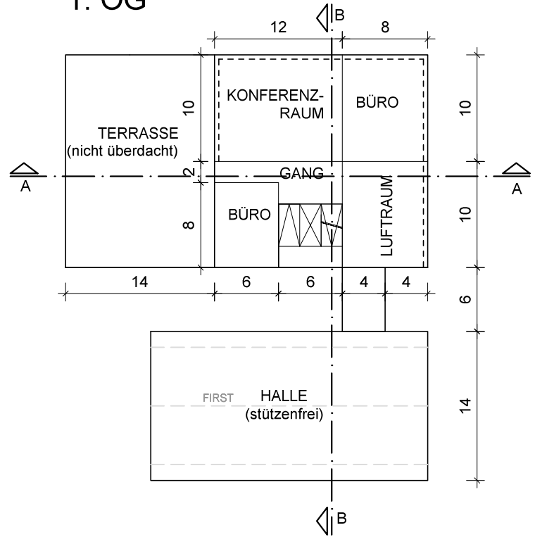
1. OG
