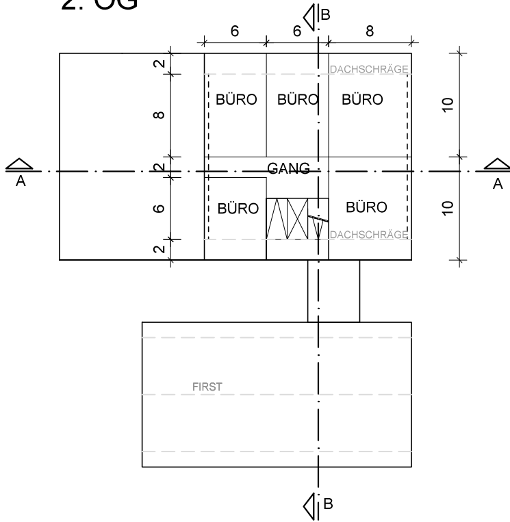
2. OG
