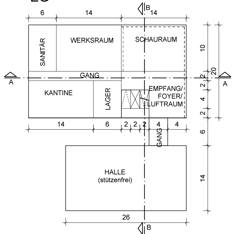
EG
