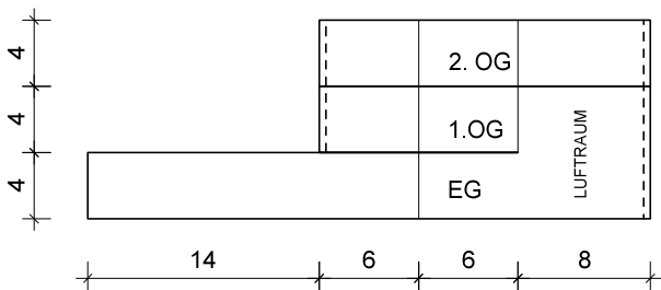
SCHNITT B-B
